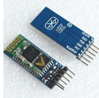
Figure4 Bluetooth Module (HC-05)
